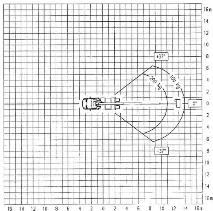
Abstützung in Fahrzeugbreite, Breite: 2,15 m
