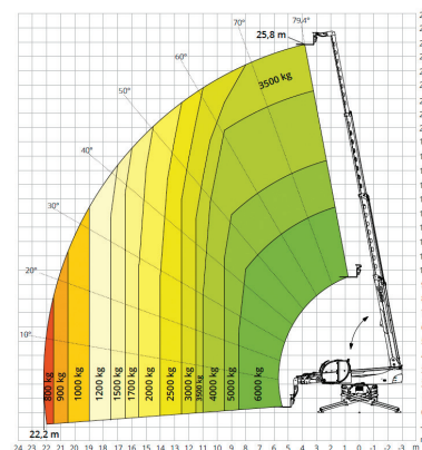
Ausgefahrene Stützen 360 Grad
