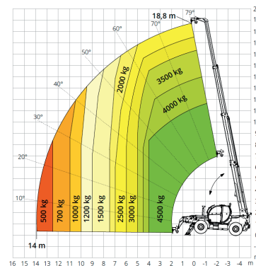
Lastdiagramm mit LASTHAKEN 5.000 kg ATT-05-014
