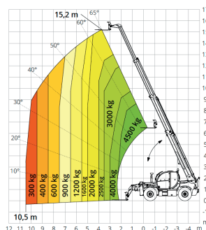
Lastdiagramm FRONTAL AUF REIFEN ATT-03-042
