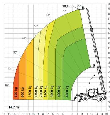
Lastdiagramm mit AUSGEFAHRENEN STÜTZEN ATT-03-042
