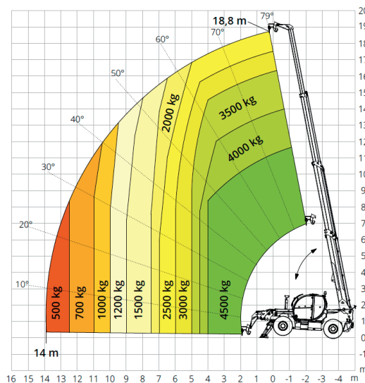
Lastdiagramm mit LASTHAKEN 5.000 kg ATT-05-014
