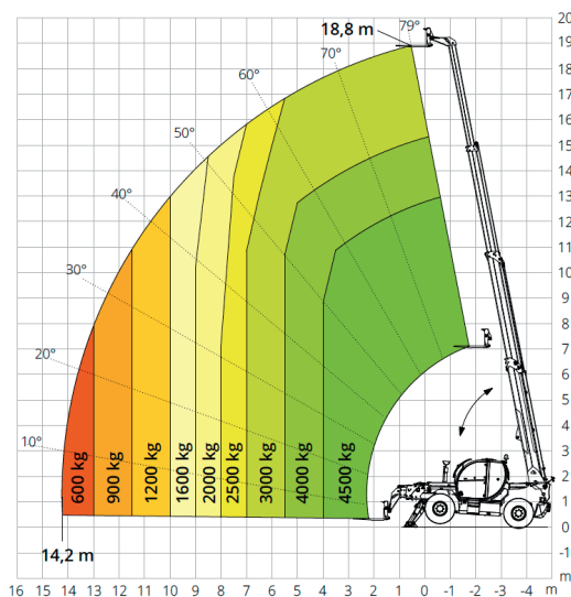
Lastdiagramm mit AUSGEFAHRENEN STÜTZEN ATT-03-042
